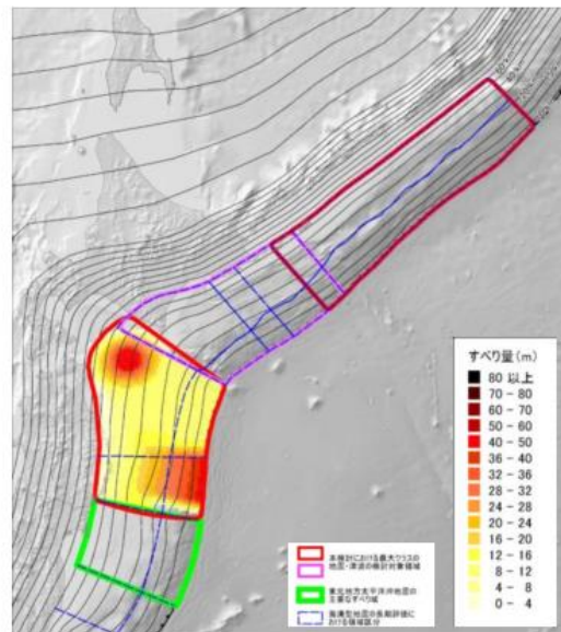
日本海溝（三陸・日高沖）モデル（Mw 9.1）
