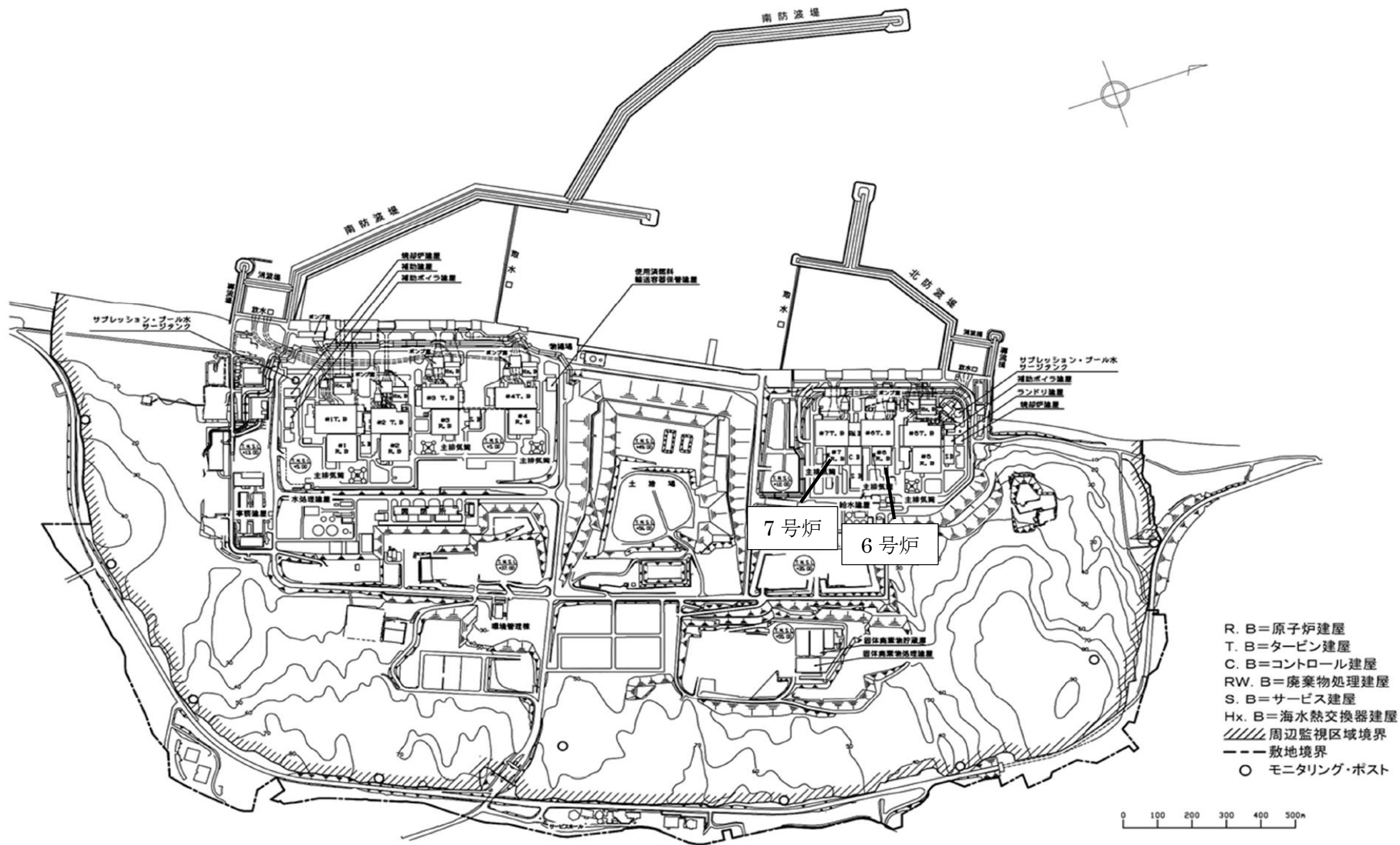
参考図 発電所全体配置図
