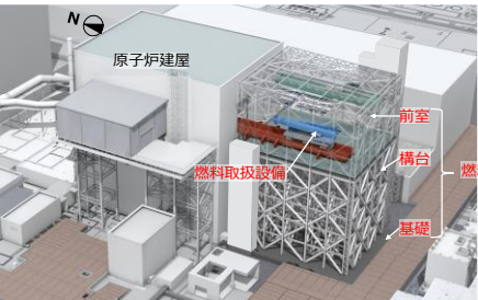
燃料取り出し工法（イメージ図）
