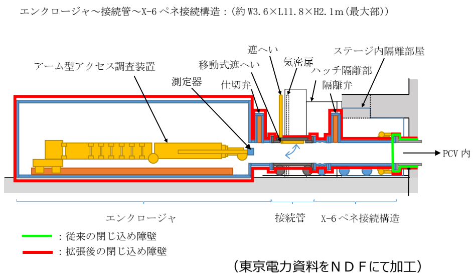
図 X-6 ペネ エンクロージャ等 構造概略図
