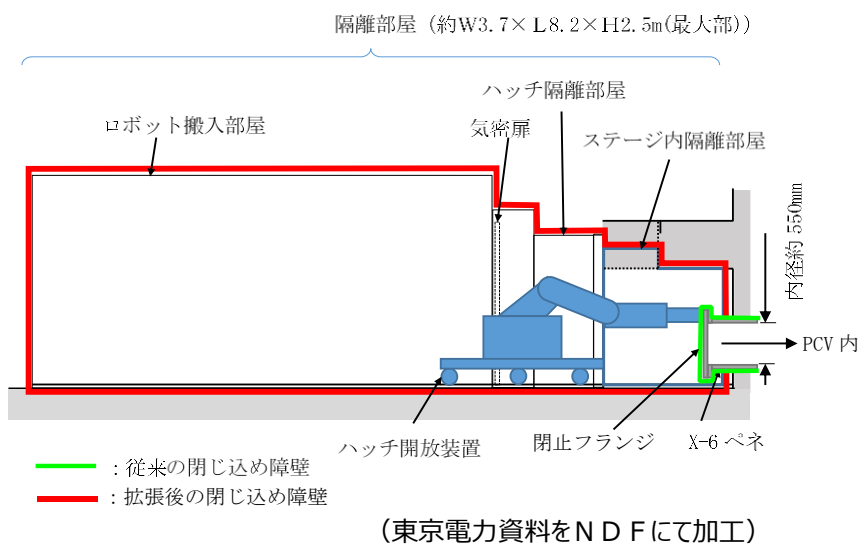
図 X-6 ペネ 隔離部屋 構造概略図
