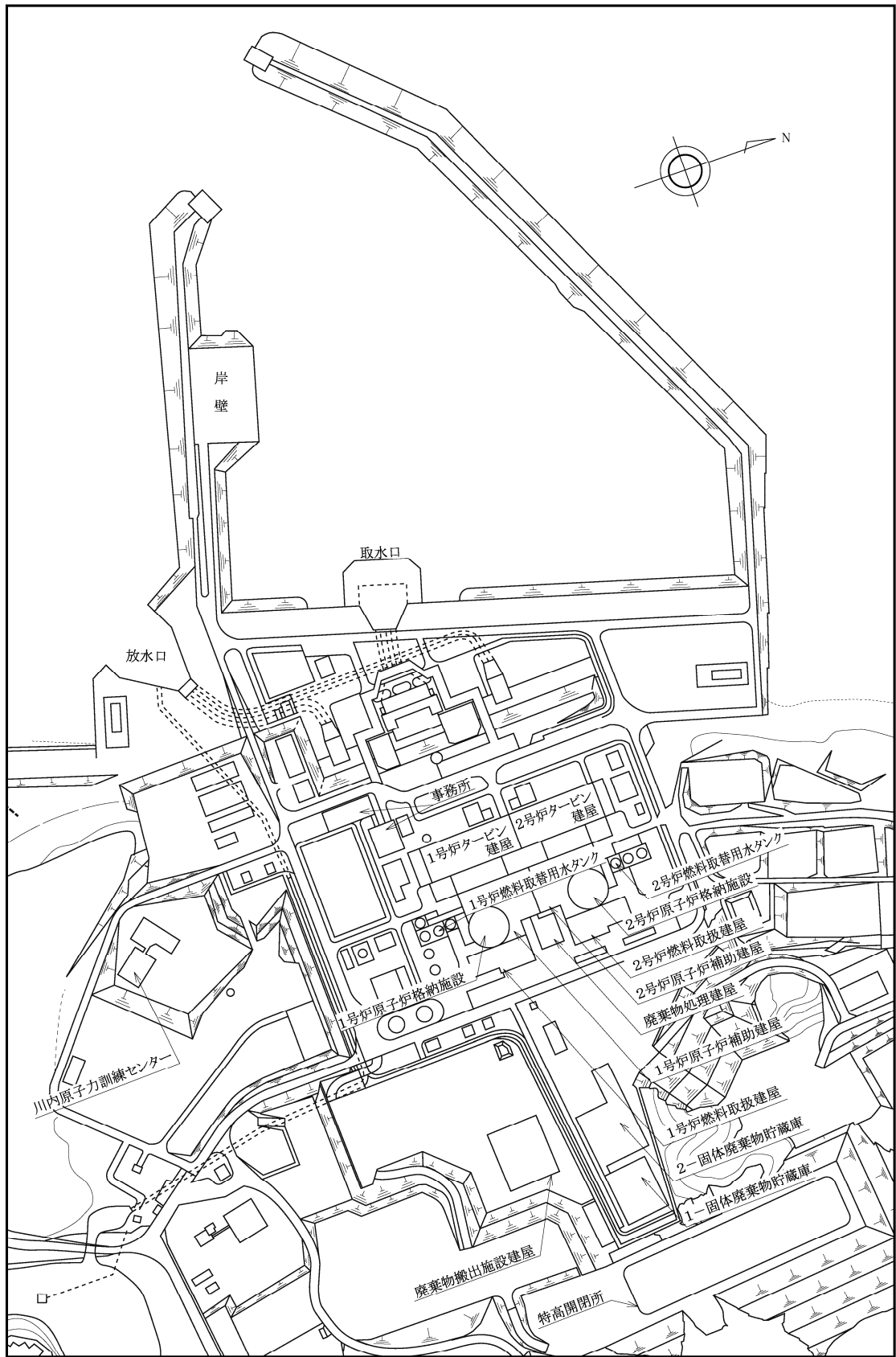
参考図 発電所全体配置図
