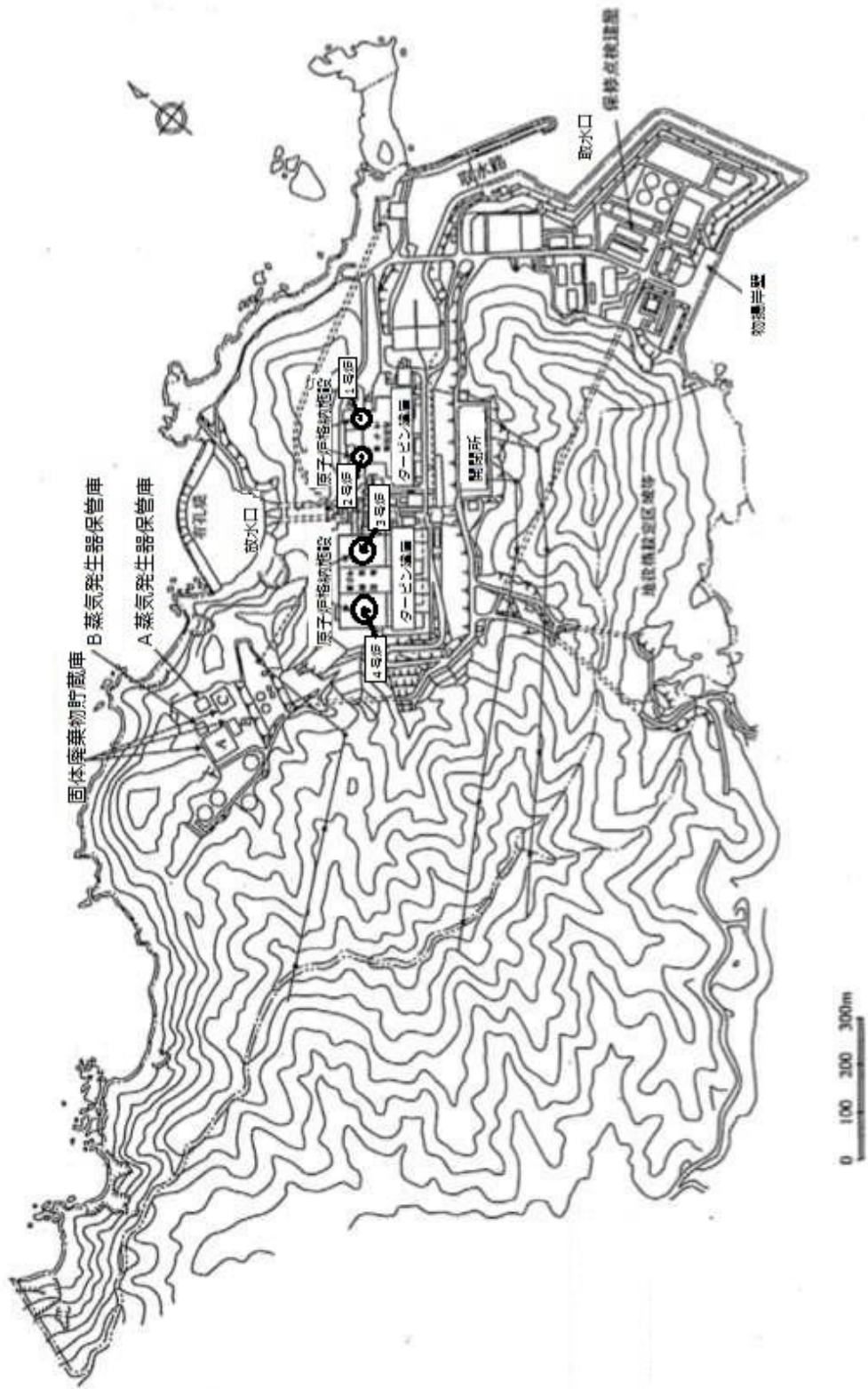
参考図 発電所全体配置図
