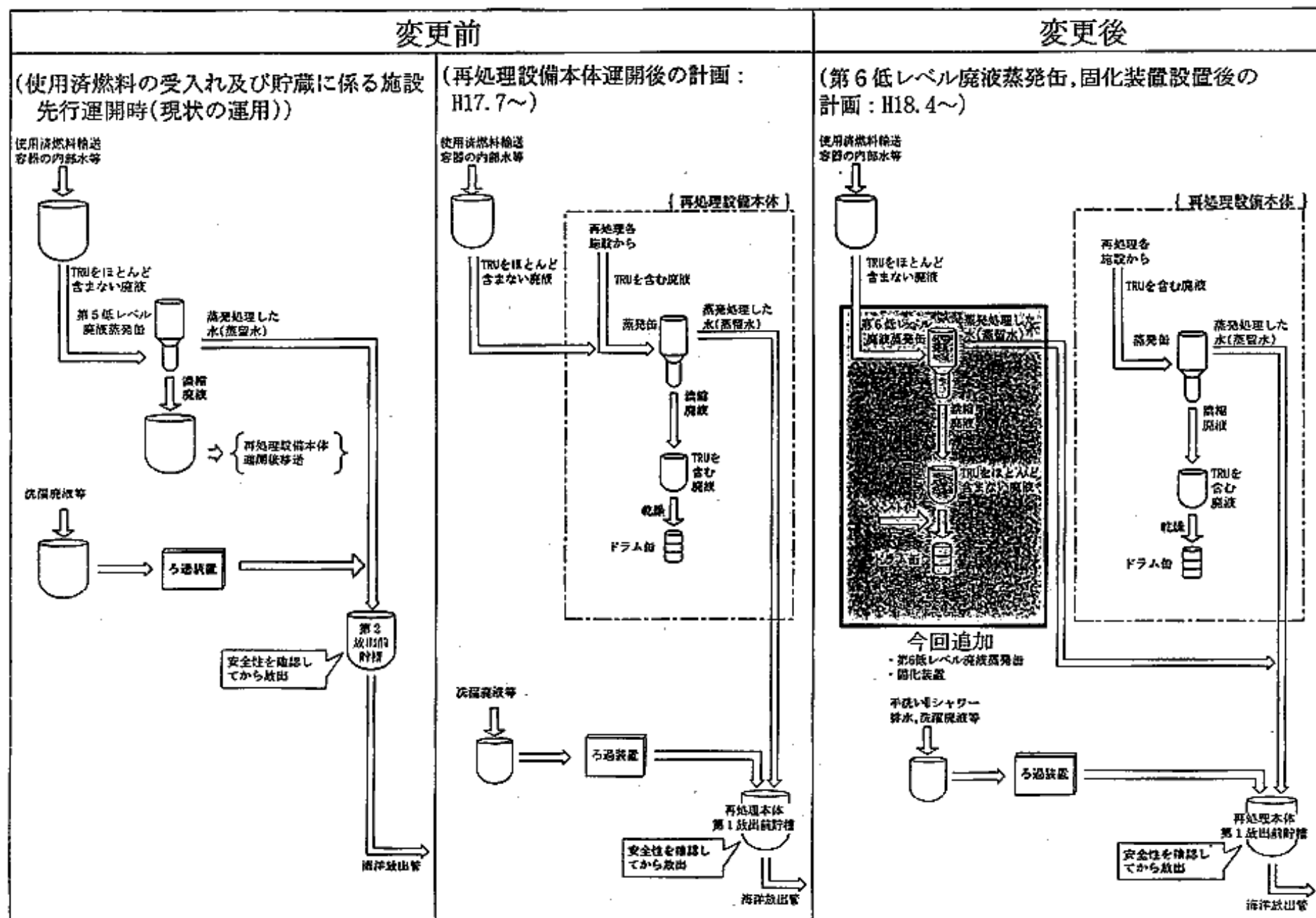
第2図 使用済燃料受入れ・貯蔵建屋の低レベル廃液処理の変更概要
