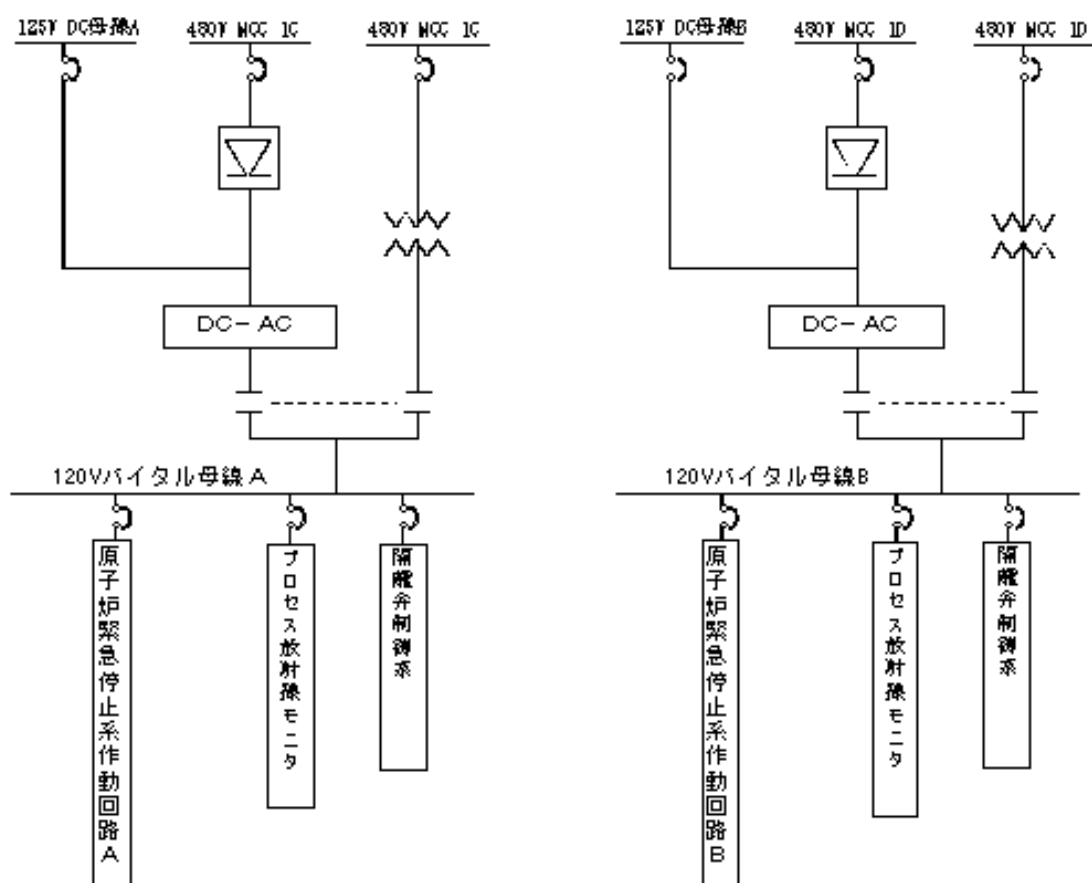
第6図 計測制御用電源系統図（変更案）
