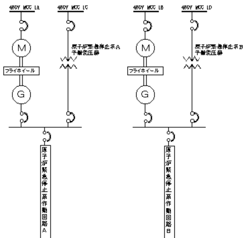
第5図 原子炉緊急停止系作動回路MGセット電源構成（現状）
