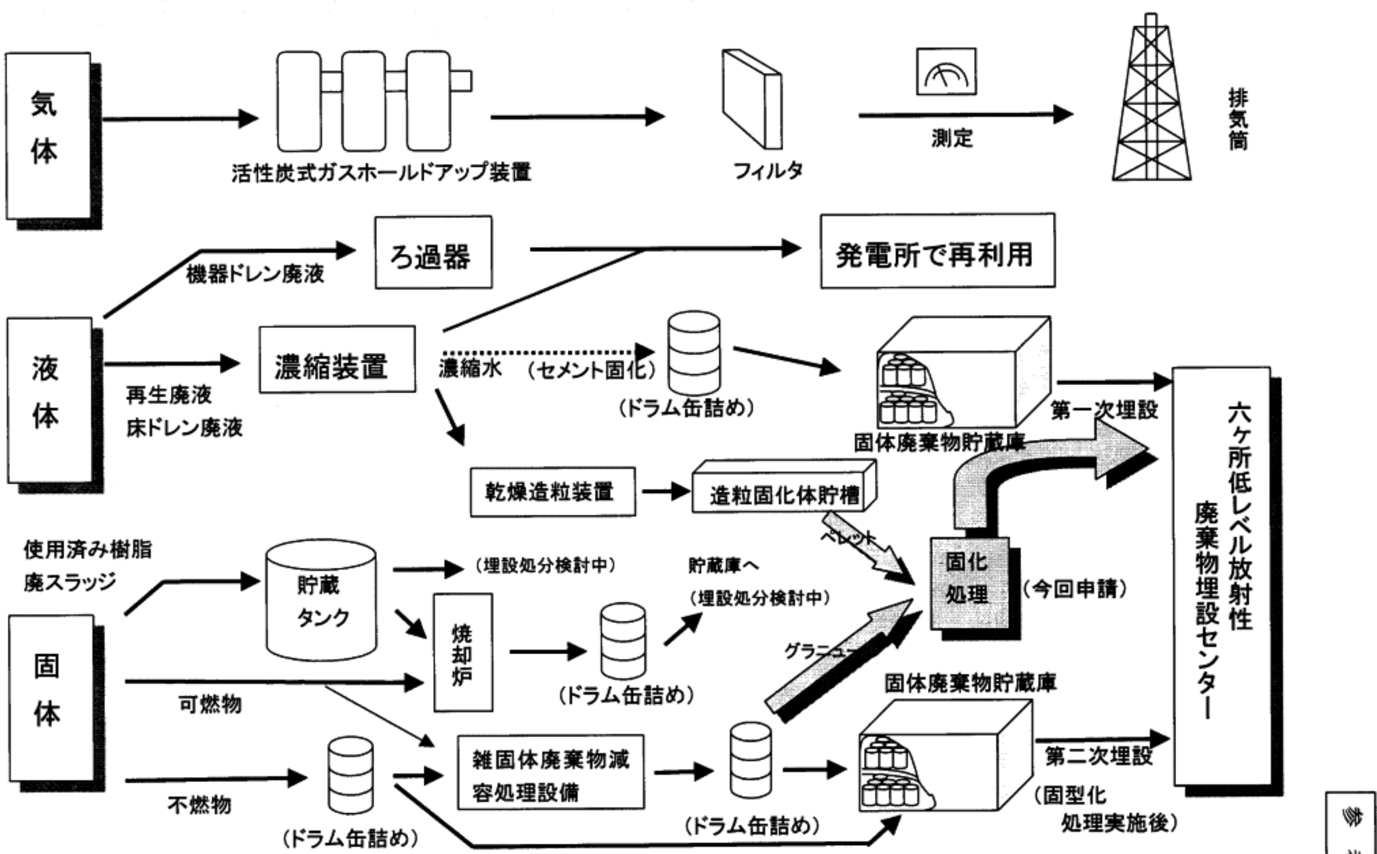
放射性廃棄物処理処分フロー図
