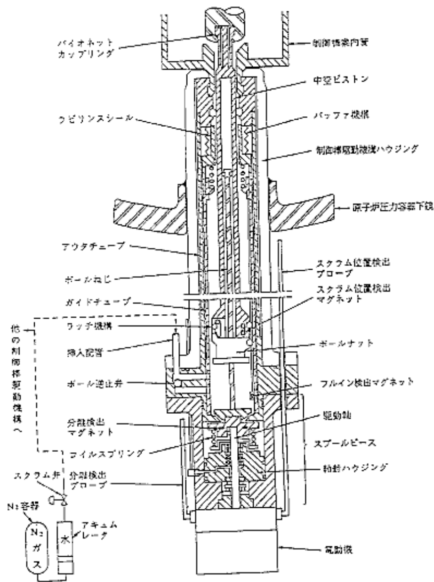
制御棒駆動機構（変更前）
