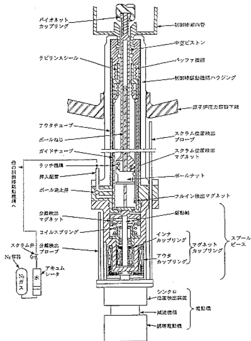
制御棒駆動機構（変更後）
