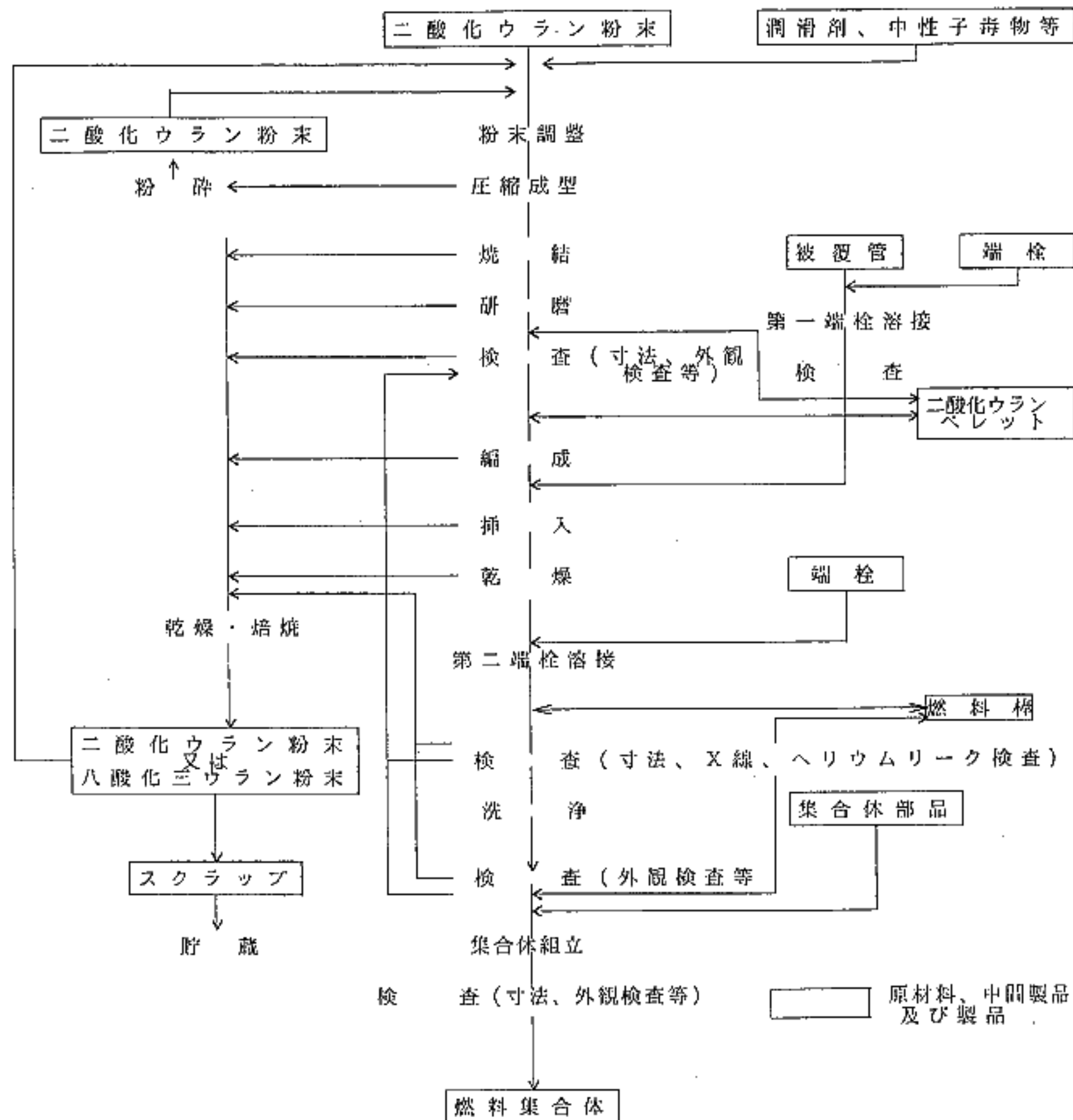
軽水炉用燃料製造工程図
