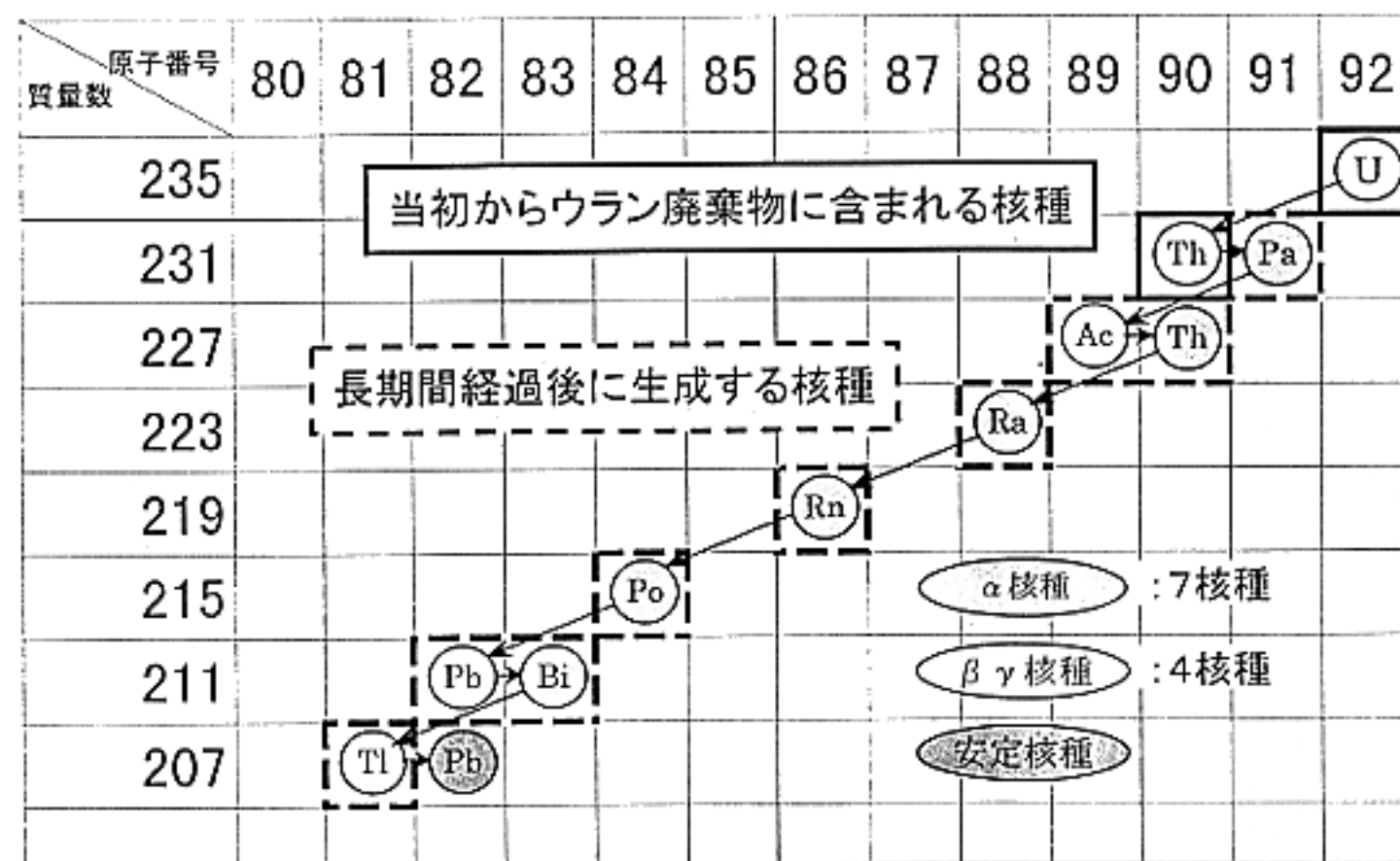
図 2 235-Uの崩壊系列
