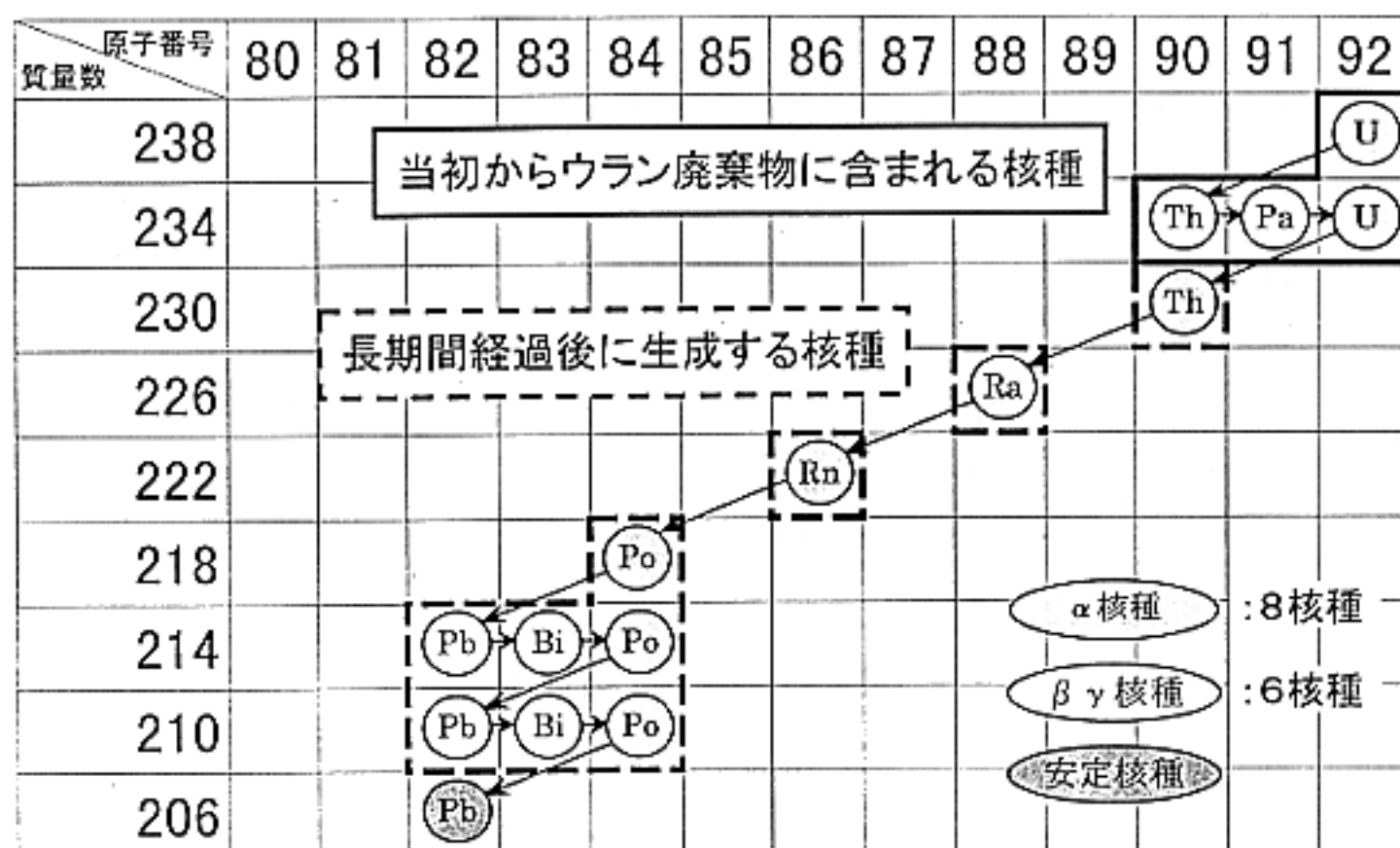
図 1 238-Uの崩壊系列
