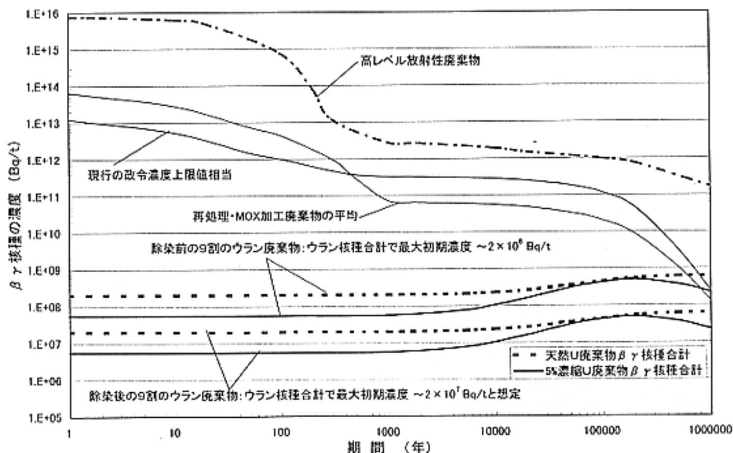
図2 ウラン廃棄物の \beta 、 \gamma 核種濃度の経時変化（他放射性廃棄物との比較）
