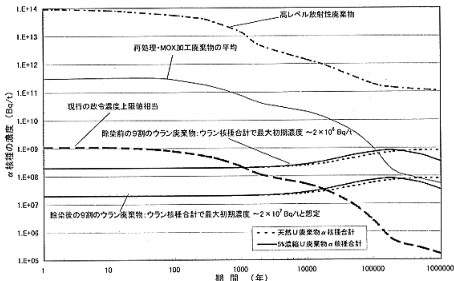
図1 ウラン廃棄物の \alpha 核種濃度の経時変化（他放射性廃棄物との比較）
