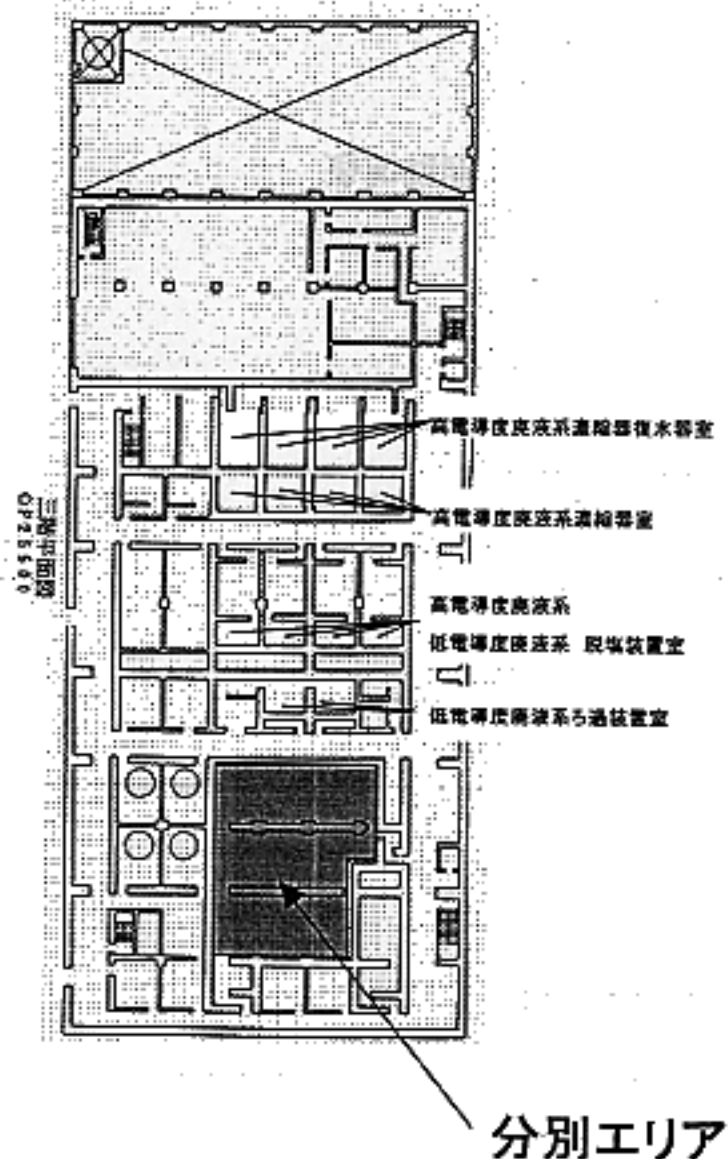
1号及び2号炉廃棄物処理建屋 3階
