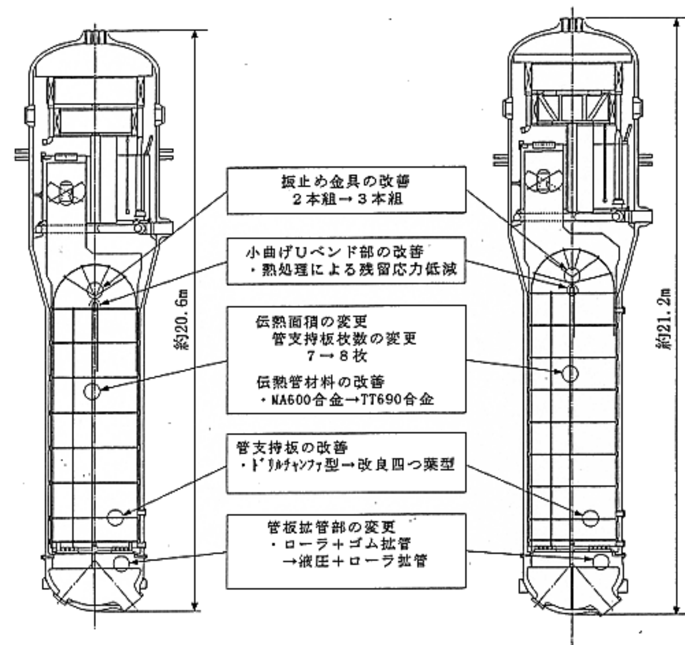
取替用蒸気発生器（54F型）
