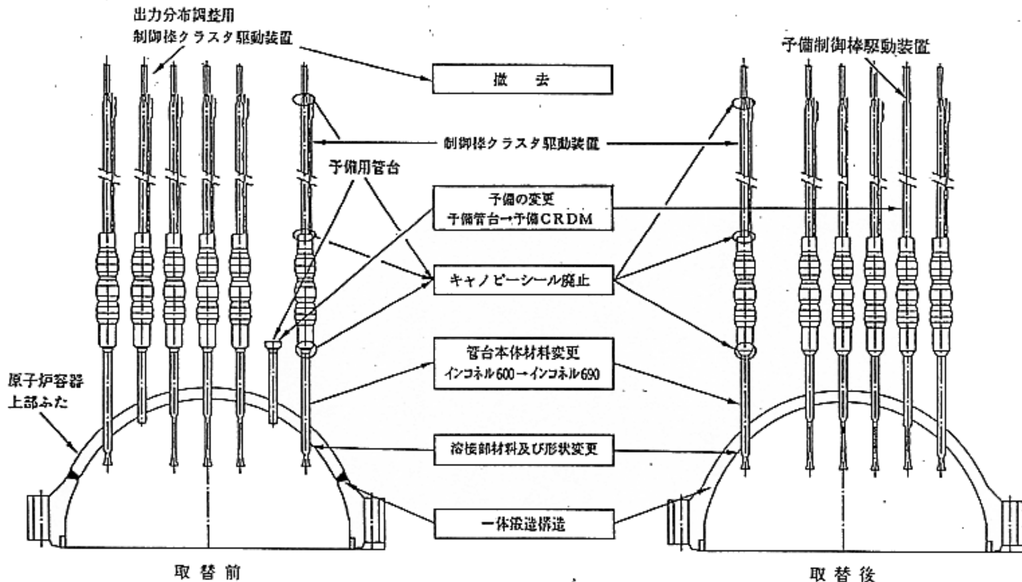
第1図 原子炉容器上部ふたの新旧比較
