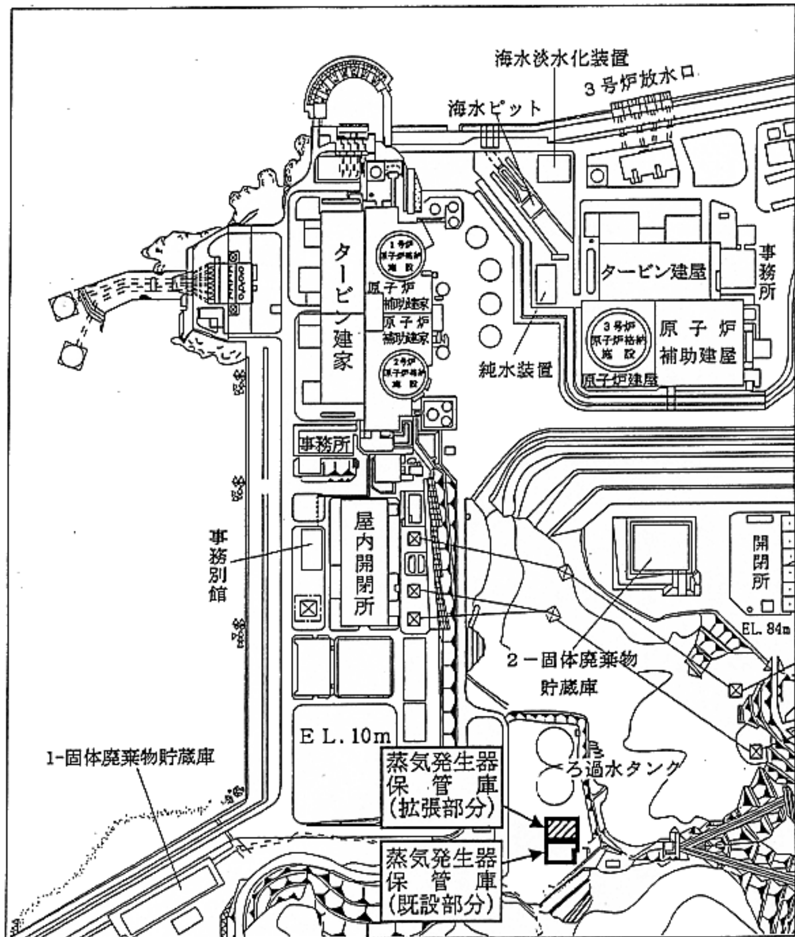
第3図 蒸気発生器保管庫の設置場所
