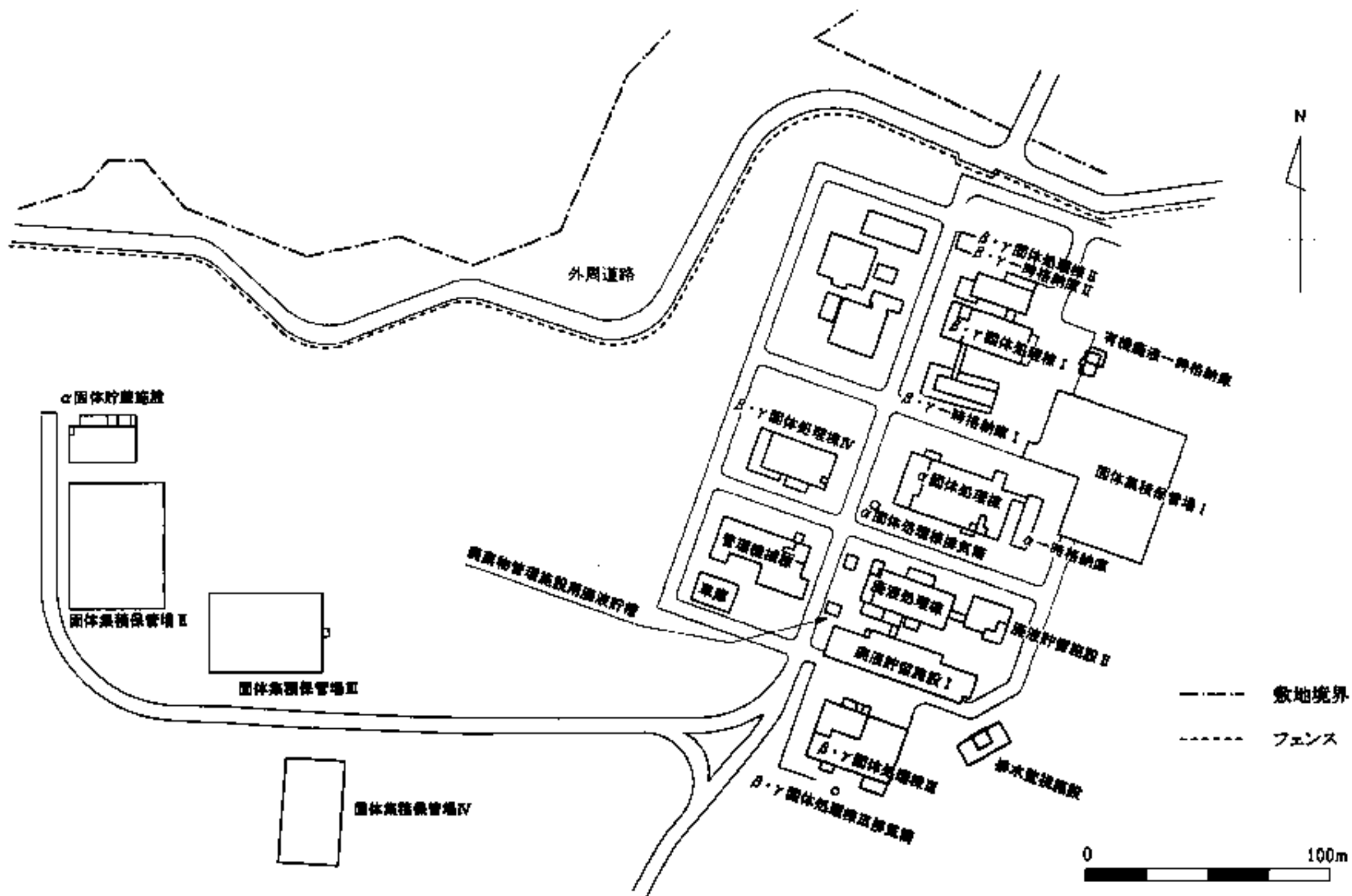
廃棄物管理施設配置図
