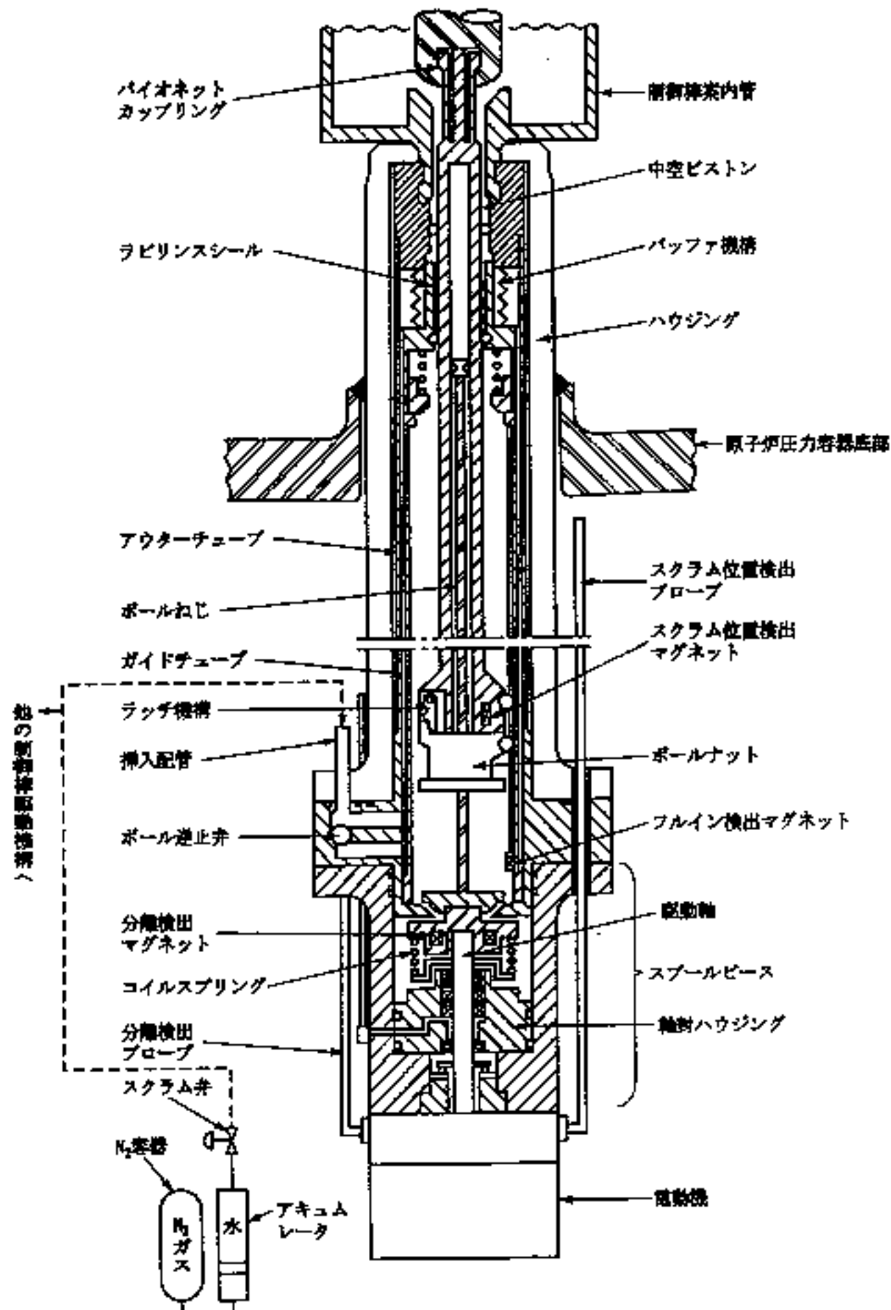
第10図 制御棒駆動機構構造概要図
