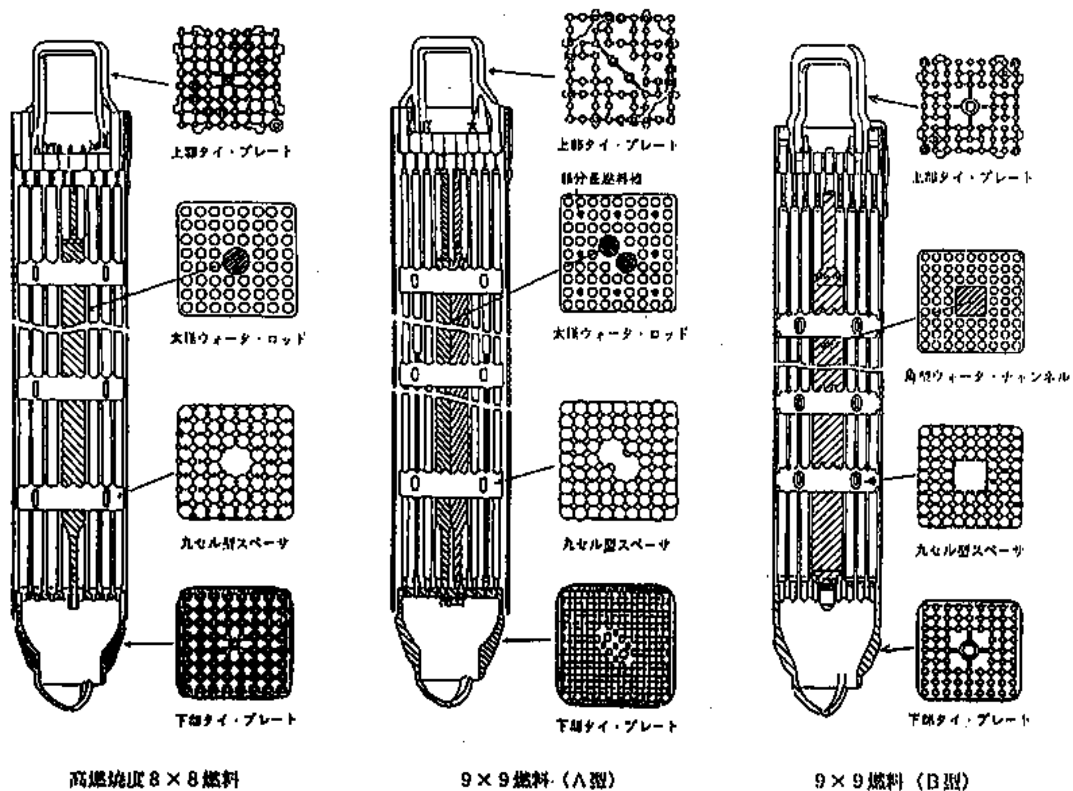
第1図 燃料集合体の主要構造の比較
