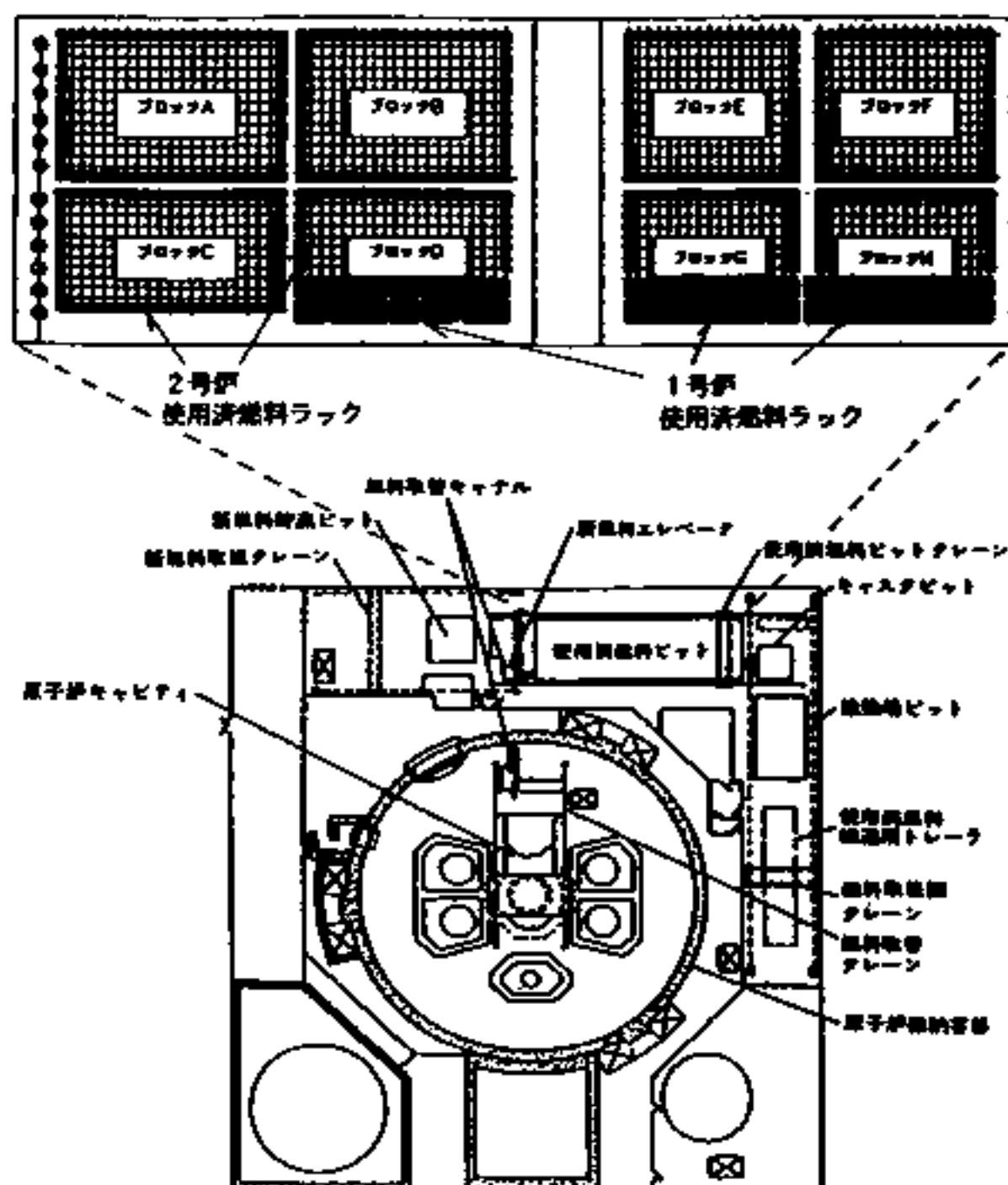
使用済燃料ビットのラック配置図
