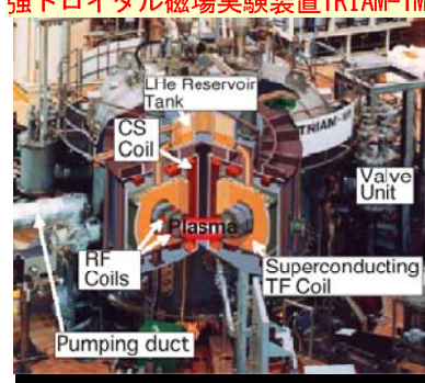
強トロイダル磁場実験装置TRIAM-1M
