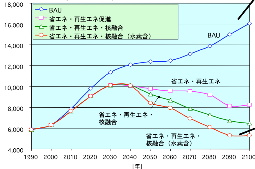
CO2排出量(炭素換算百万トン)
