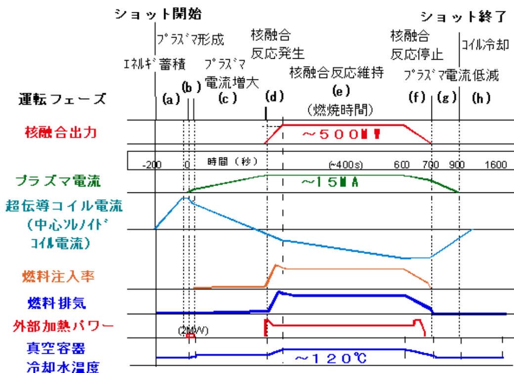
ITER 標準運転モードの代表例
