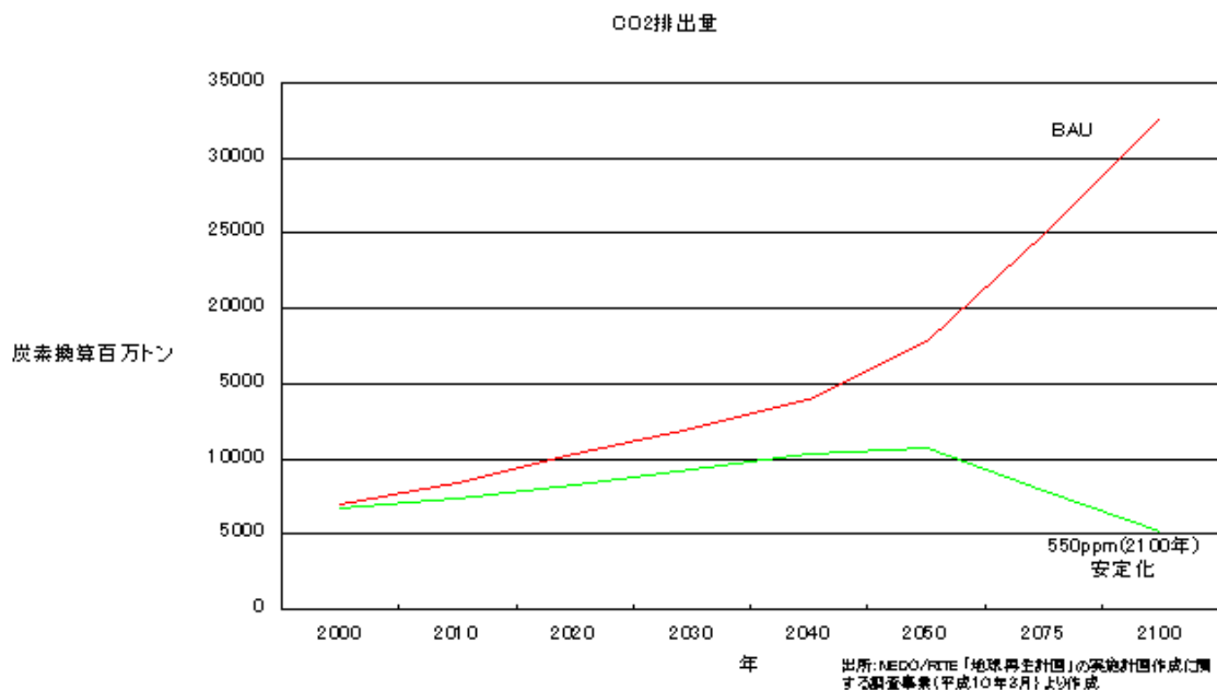
図3 CO 2 排出量
