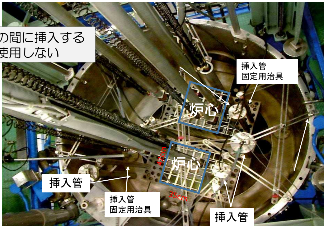
図1 軽水減速炉心（2分割炉心）
