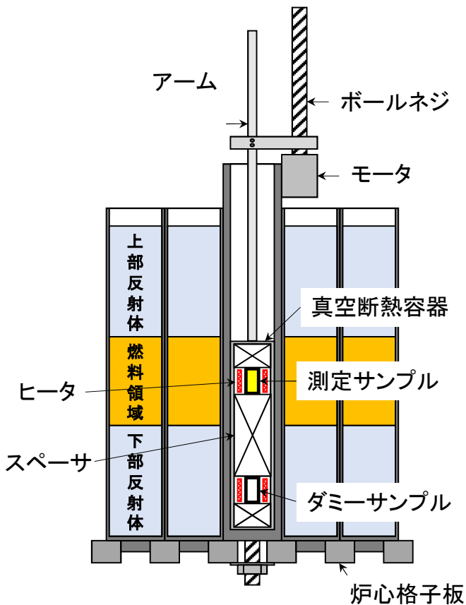
図2 パイルオシレータの概念図 （炉心を横から見た断面図）
