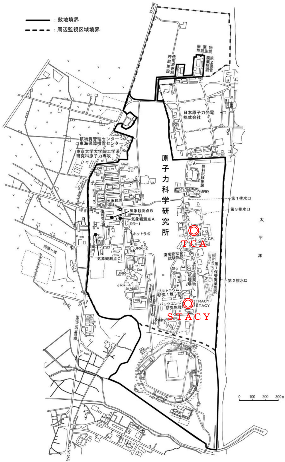
参考図 原子炉施設の位置図
