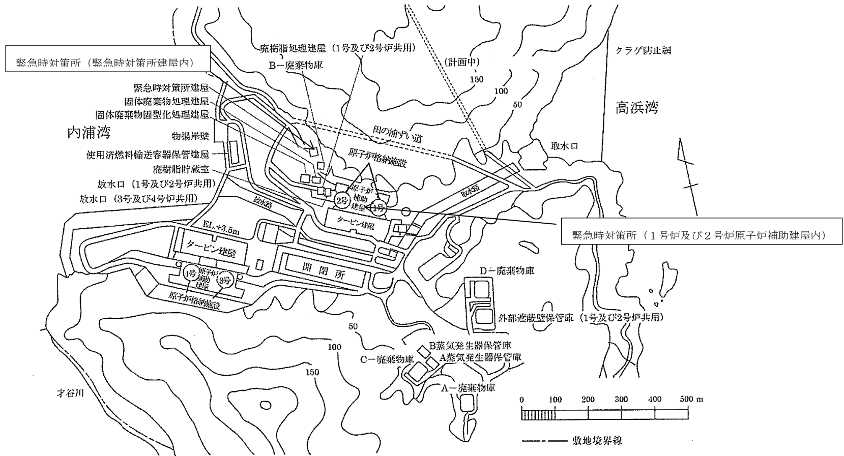
参考図 発電所全体配置図
