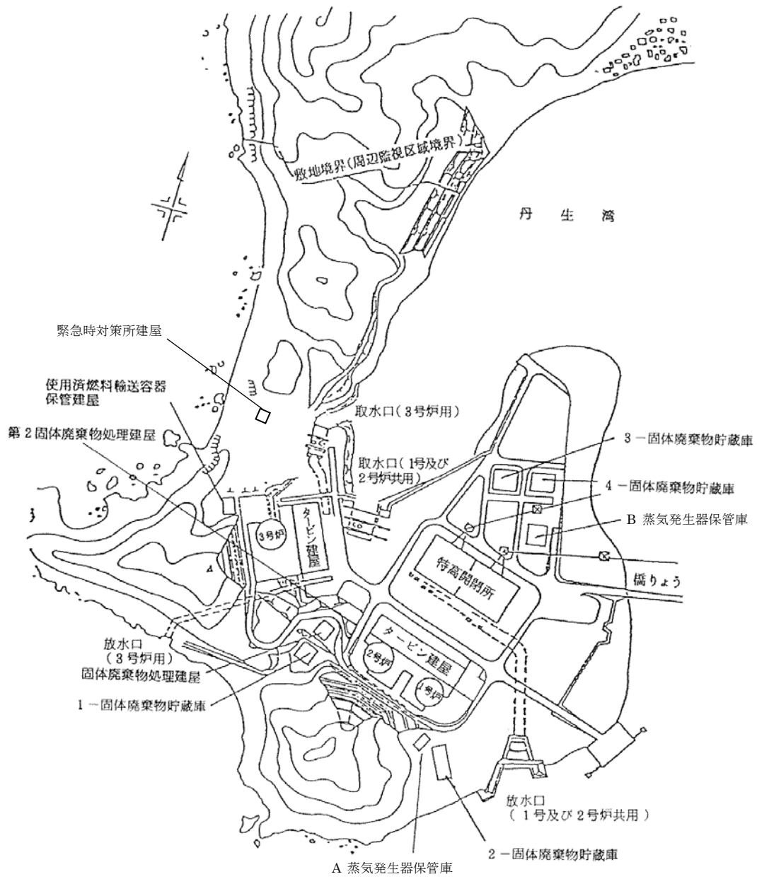
参考図 発電所全体配置図
