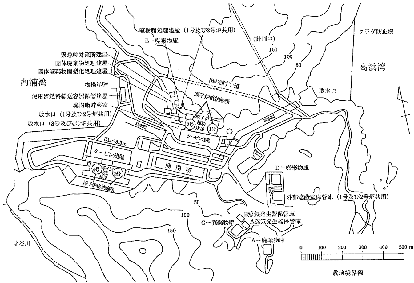
参考図 発電所全体配置図
