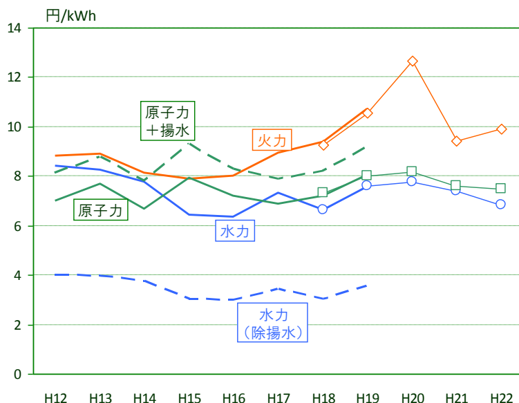
図3-8 報酬率を用いた発電コスト試算（大島：平成19年度まで、筆者ら：平成18～22年度）
