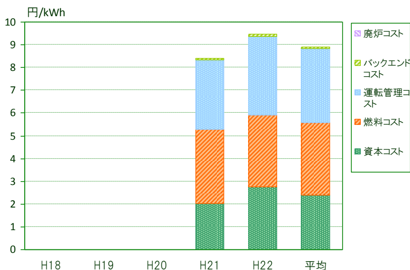
図3-7 地熱等（新エネルギー）発電コスト（電源開発を除く各社平均）
