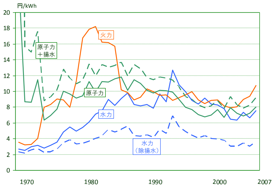
図2-2 有価証券報告書による発電単価の試算結果（大島、2010）
