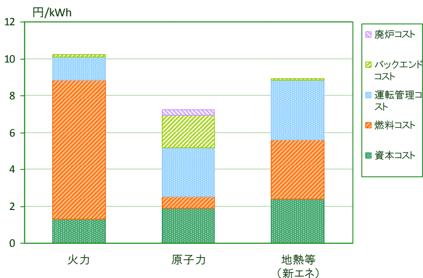
図3-1 電源別発電コスト (2006 年度～2010 年度平均)
