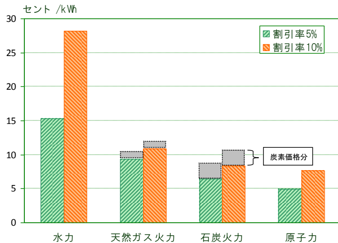
図4-1 日本を対象とした発電コスト試算結果 (OECD、2010)
