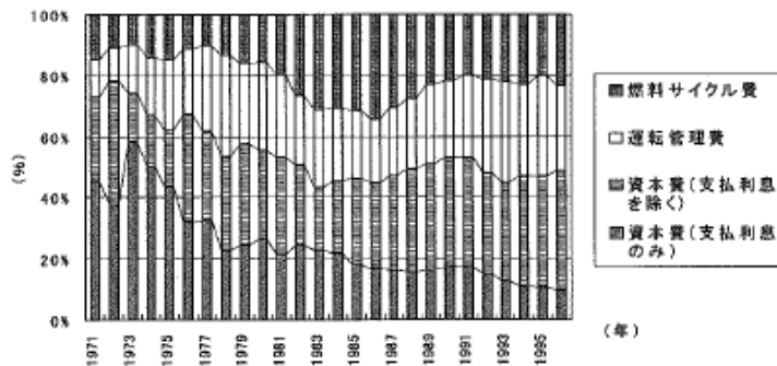
図2 財務諸表に基づく原子力発電コストの構成割合
