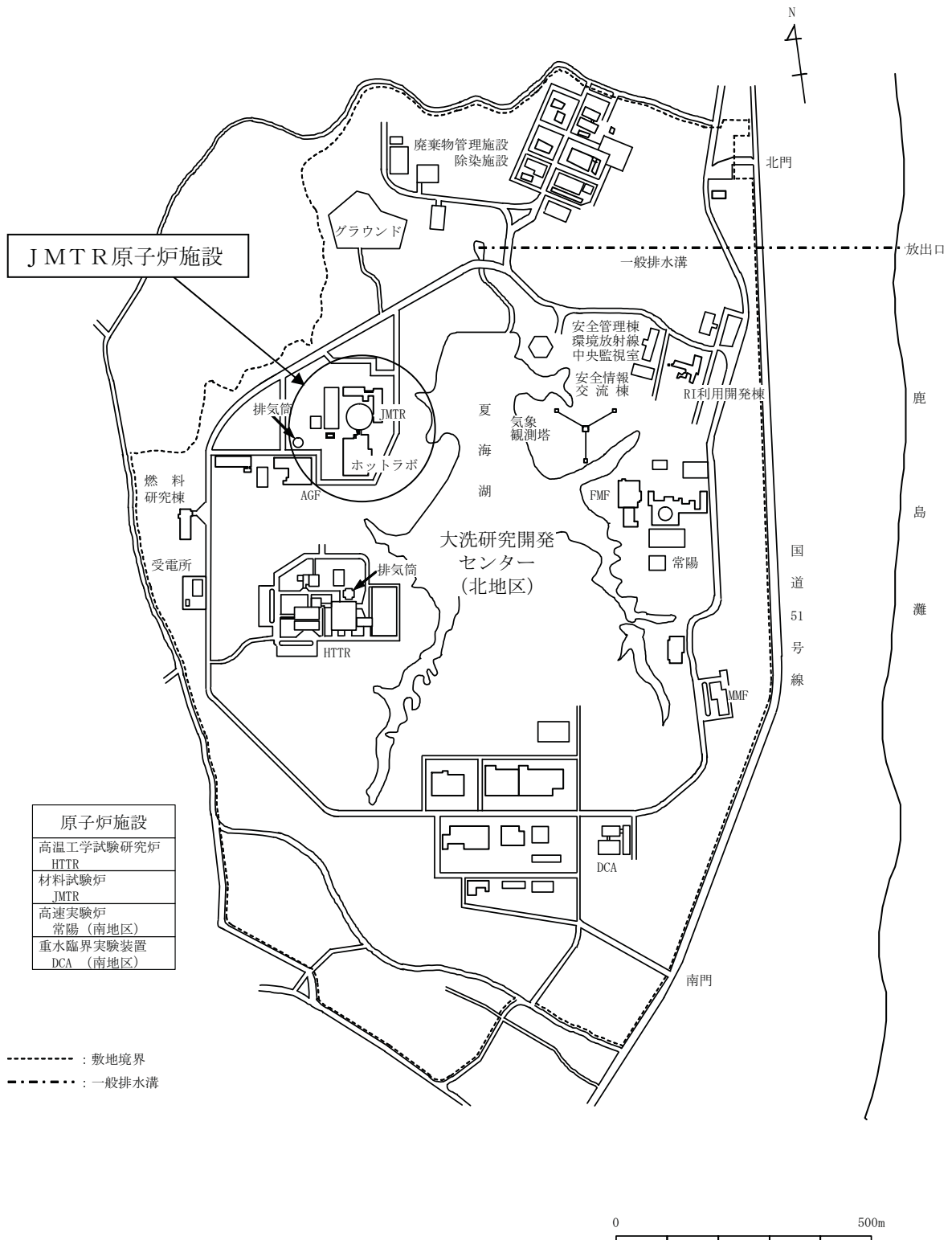
図 独立行政法人日本原子力研究開発機構 大洗研究開発センター (北地区) 配置図
