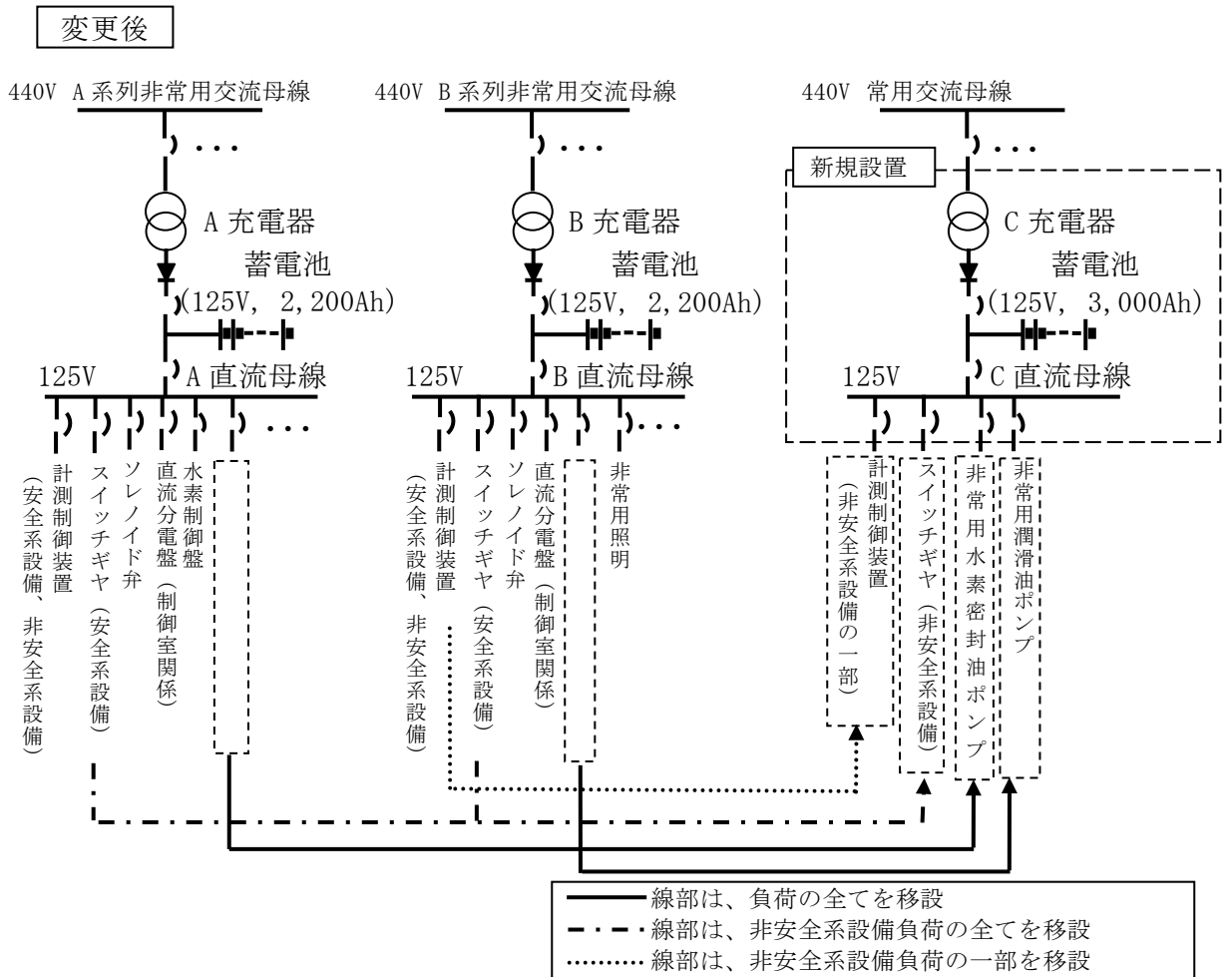
第5図 蓄電池負荷の変更概略図 (1号炉)
