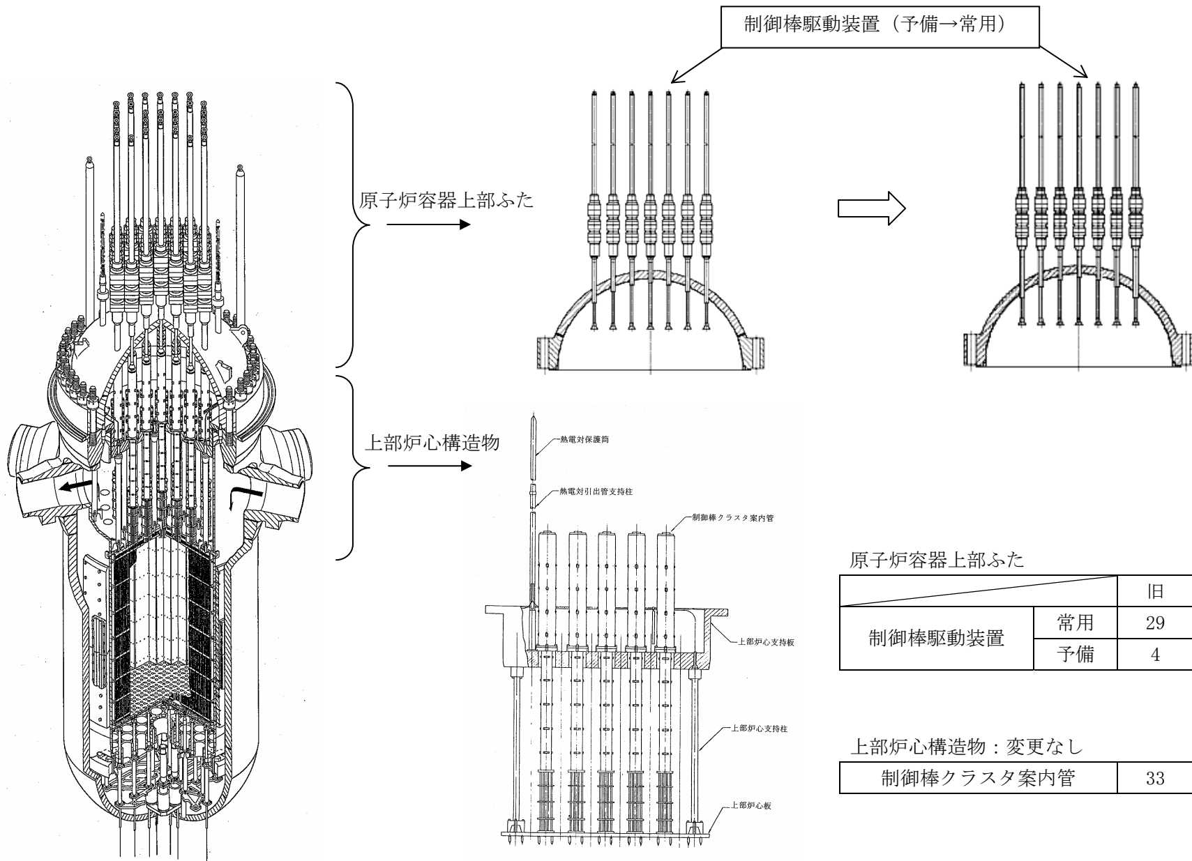
第2図 原子炉容器上部ふた並びに上部炉心構造物 概要図
