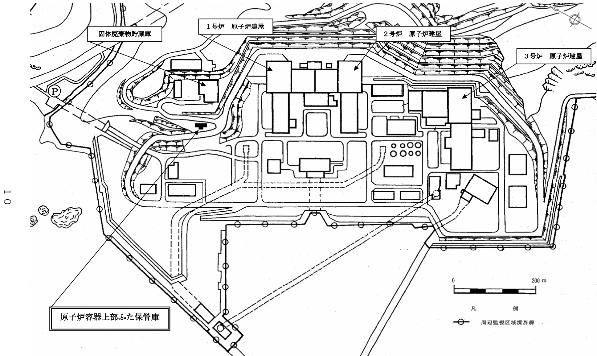
第3図 原子炉容器上部ふた保管庫増設場所
