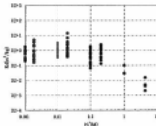
図 Na濃度とCsの単価への収着分配係数の関係(湯谷ほか, 1999, 岡山ほか, 2004)
