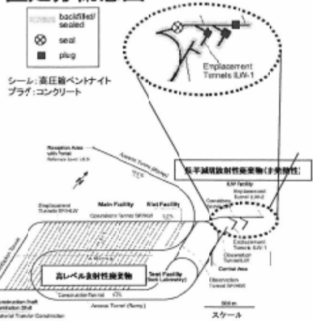
図 オパリナス粘土層における地層処分場レイアウト 出典: Nagra NTB 02-05: Project Opalinus Clay
