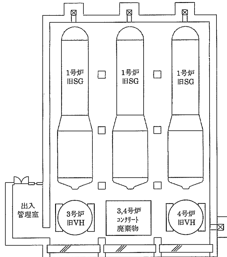
B 蒸気発生器保管庫
