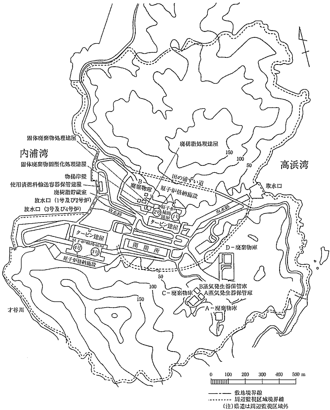
第1図 発電所全体配置図
