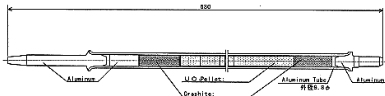
図1 Al 被覆燃料棒
