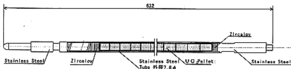
図2 SUS 被覆燃料棒
